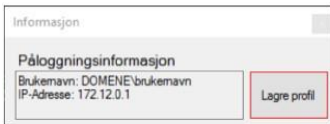
Figur 3 - Påloggingsinformasjon
