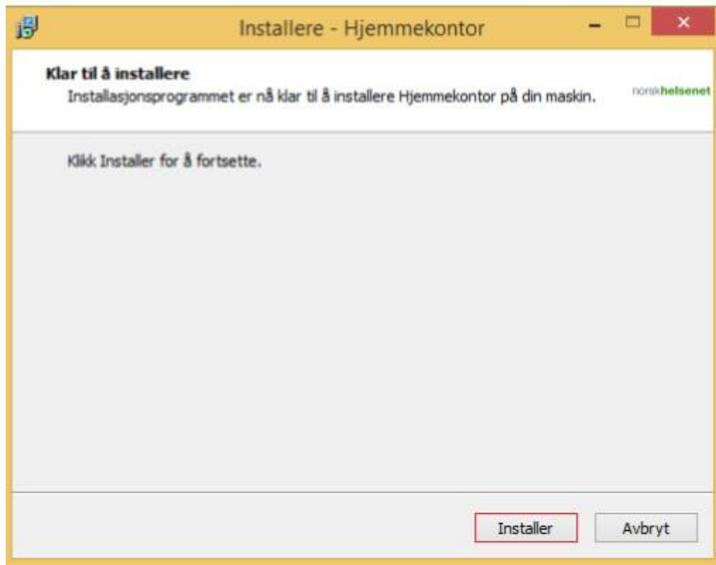
Figur 2 – Installere
